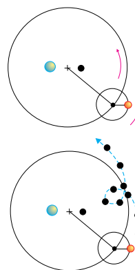
▲ Explicarea mișcărilor retrograde ale planetei cu ajutorul epiciclurilor.
