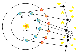
▲ Primul model, heliocentric al lui Copernic.
